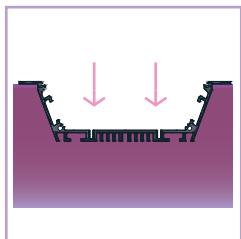
1 Empotrar el perfil en una superficie
