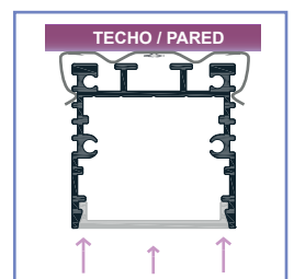
② Encajar el perfil en las grapas hasta que haga "click"
