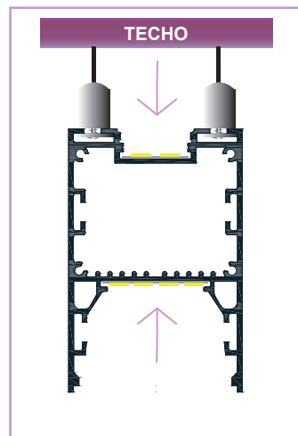
③ Pegar el adhesivo de las tiras LED al perfil
