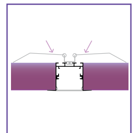
③ Dejar caer las aletas de las pinzas al empotrarlo y encajar el perfil
