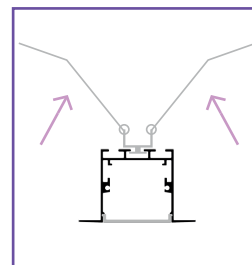
② Abrir las aletas de las pinzas para empotrarlo
