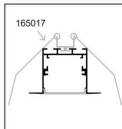
① Colocar las pinzas en el perfil
